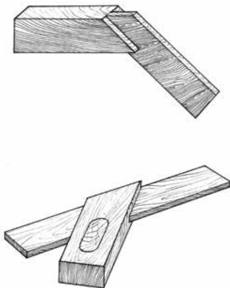
Rys. 2.4. Kątownik ukośny - węgielnica uciowska – giermas .
