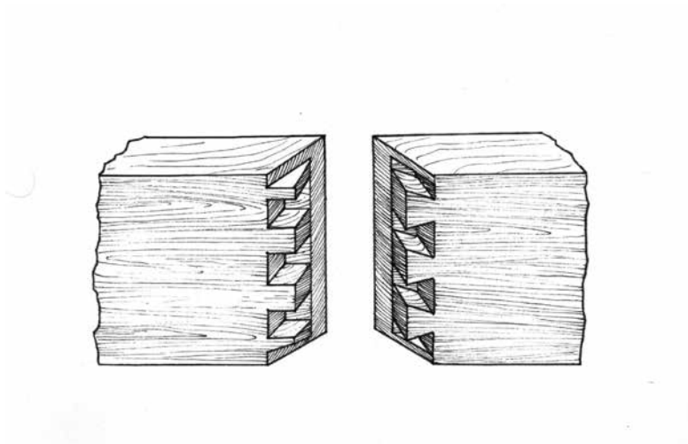
Rys. 3.22. Zazębienie (cynki) kryte na ucios – gierungcynki
