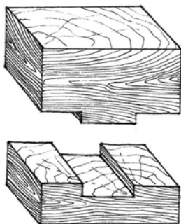
Rys. 3.16. Połączenie krzyżowe – wcios krzyżowy.
