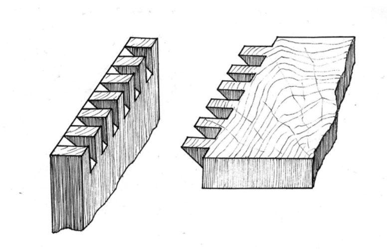
Rys. 3.23. Zazębienie na ucios częściowo kryte.
