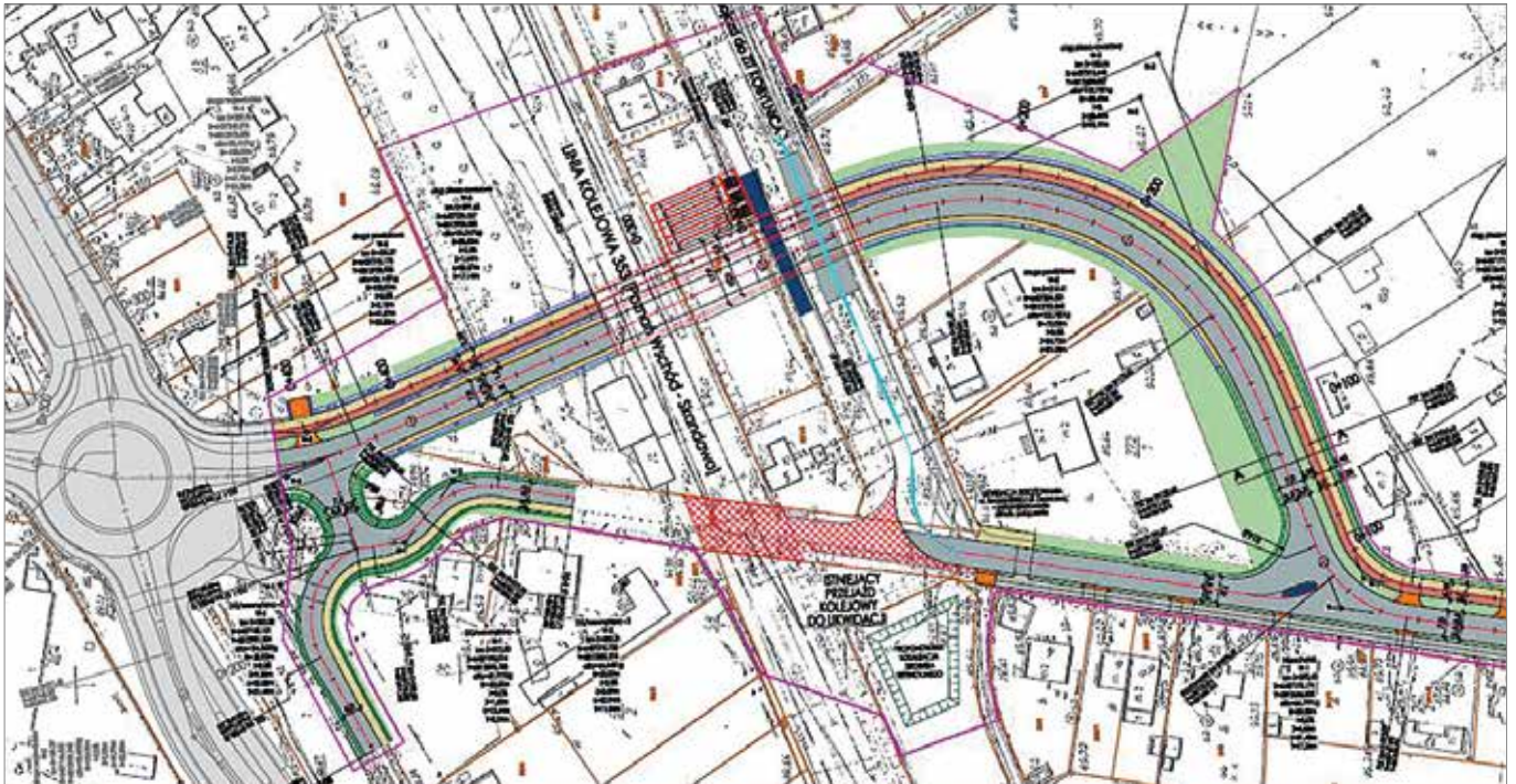
Budowa tunelu w Kobylnicy wraz z przebudową skrzyżowania z ul. Poznańską
