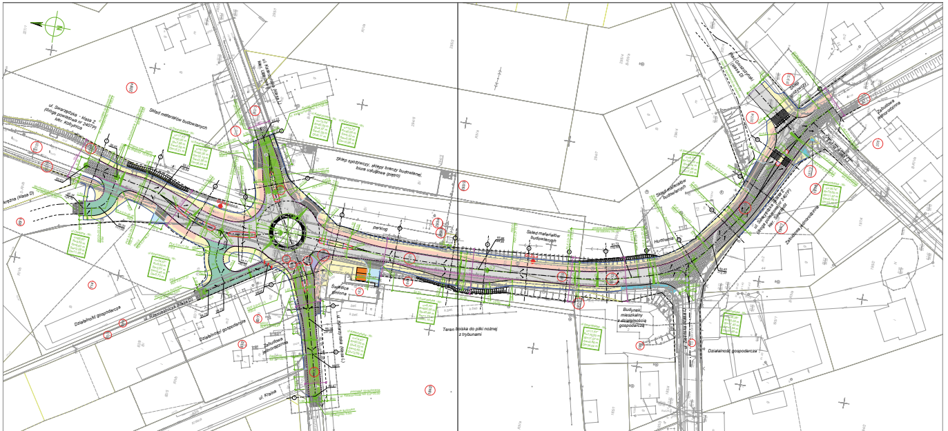
Koncepcja budowy ronda w rejonie ulic Swarzędzka – Katarzyńska
